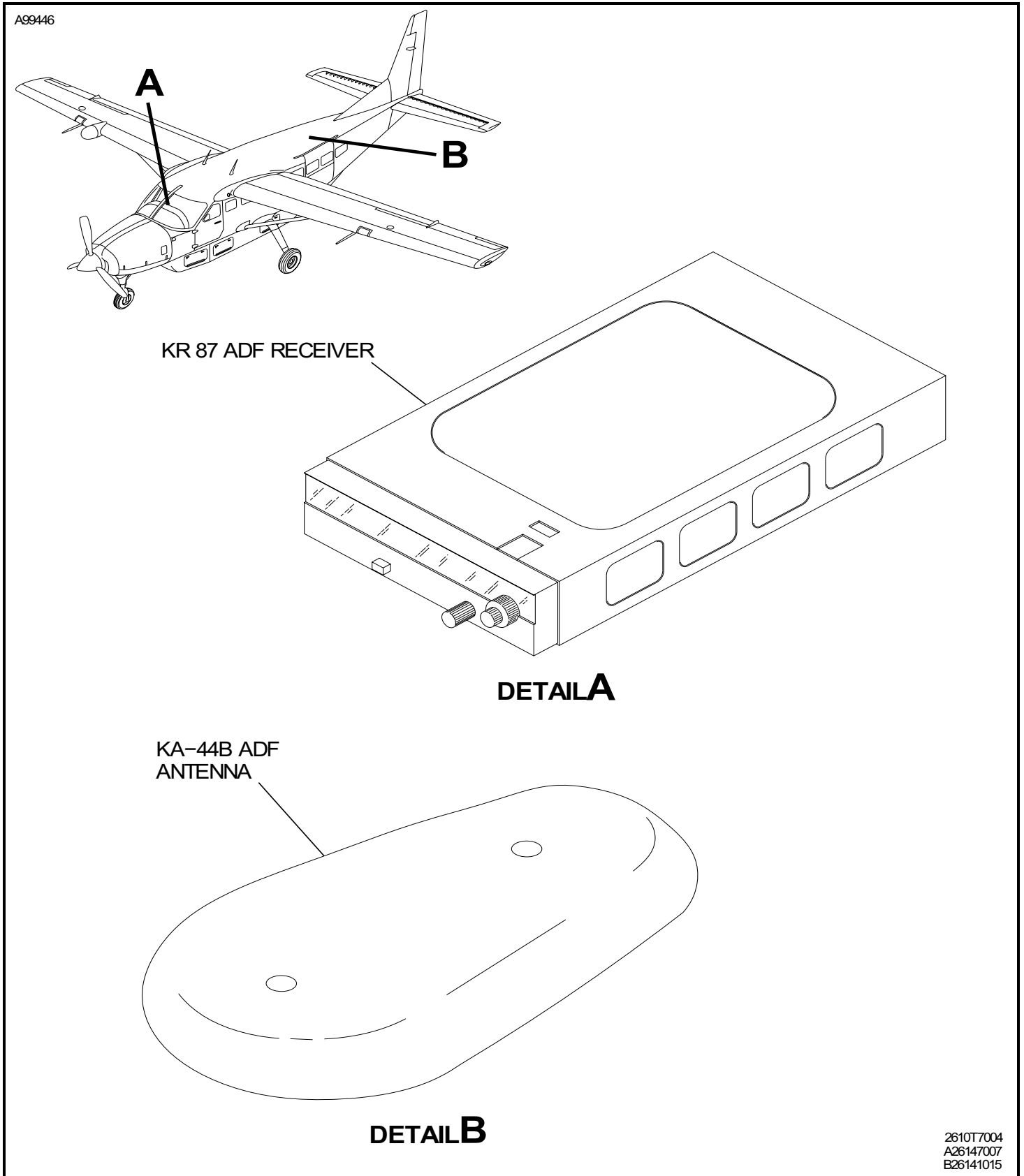
Figure 1 : Sheet 1 : Bendix/King KR 87 ADF System
